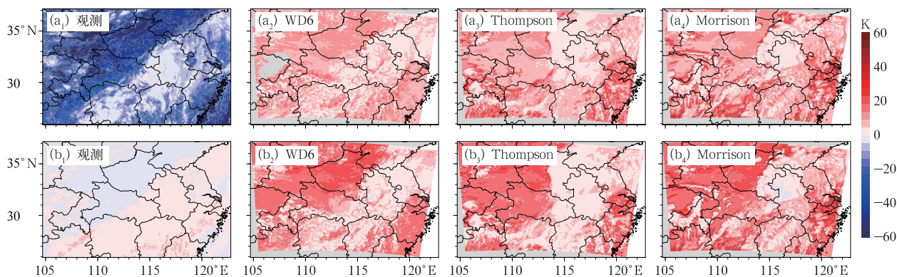
图 9 2016 年 7 月 1 日 07 时葵花 8 卫星观测及三种云微物理方案模拟的两个通道亮温差值
