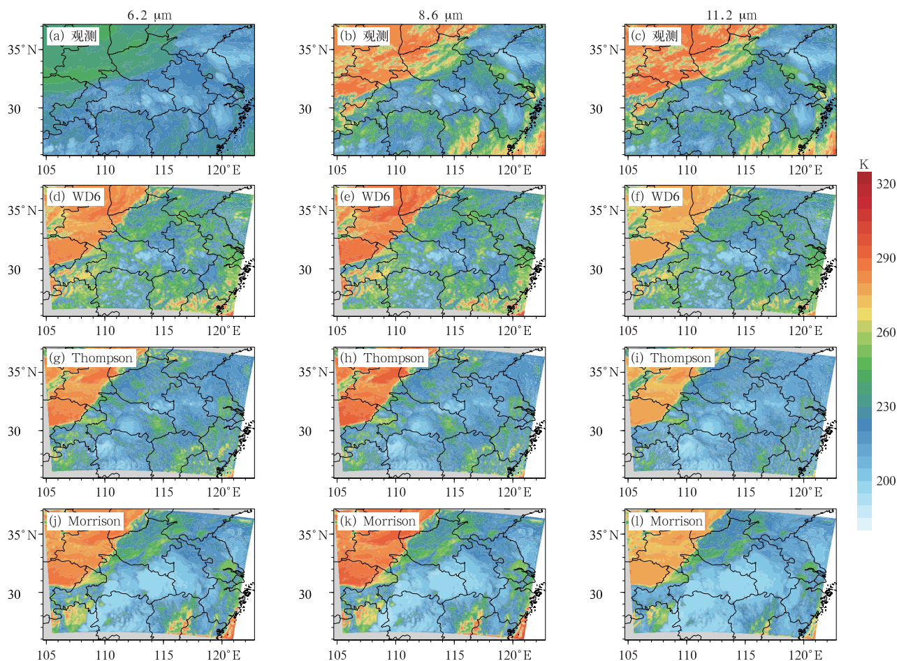
图7 2016年6月30日18时葵花8卫星观测及三种云微物理方案模拟的三个通道亮温
