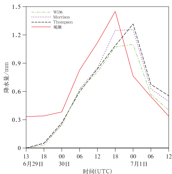
图5 2016年6月29日至7月1日观测与模拟的面积平均小时降水量时间序列
