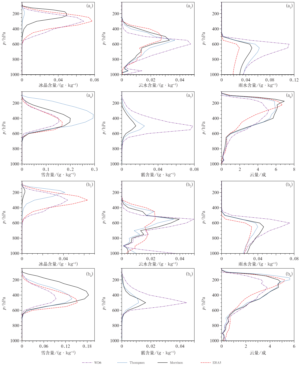
图 6 2016 年 6 月 (a) 30 日 12 时各水凝物含量和云量以及 (b) 6 月 29 日 18 时至 7 月 1 日 12 时平均的水凝物含量和云量垂直廓线 Fig. 6 Vertical profiles of hydrometeor content and cloud fraction at (a) 12:00 UTC 30 June and (b) the averaged hydrometeor content and cloud fraction from 18:00 UTC 29 June to 12:00 UTC 1 July 2016
