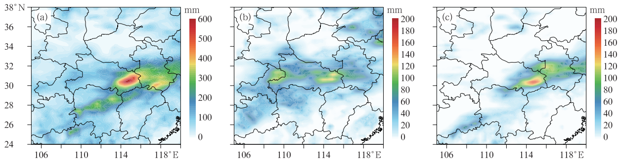
图 3 2016 年(a)6 月 29 日至 7 月 5 日累计降水量,(b)6 月 30 日、(c)7 月 1 日逐日降水量分布
