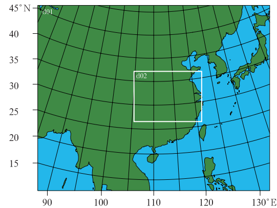
图 1 WRF 模拟的区域设置 Fig.1 Regional area for WRF simulation
