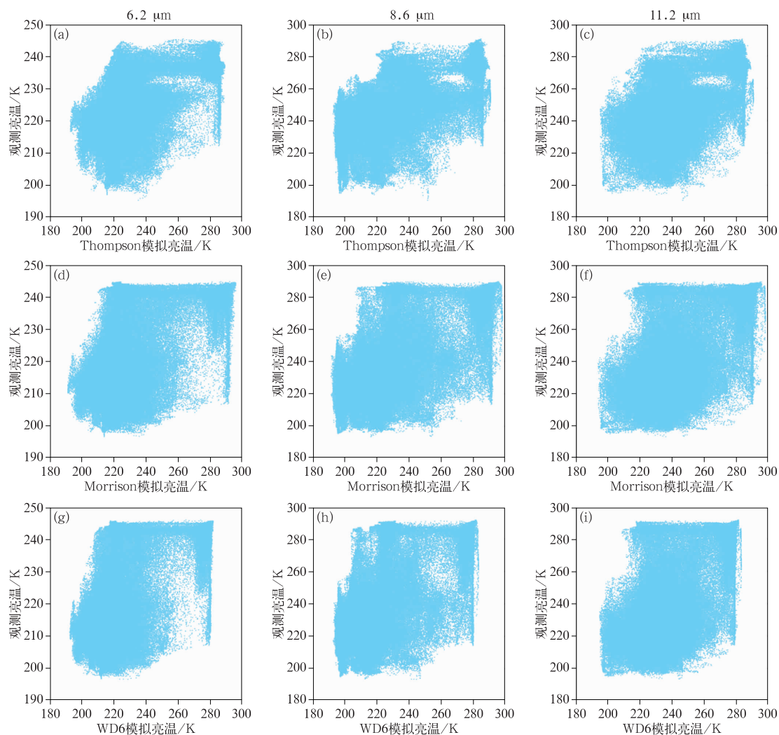
图 8 2016 年 6 月 30 日 18 时葵花 8 卫星观测及三种云微物理方案模拟的三个通道亮温散点图
