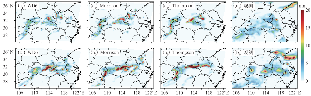
图 4 2016 年 6 月 30 日(a)12 时,(b)18 时观测及三种云微物理方案模拟的小时降水量
