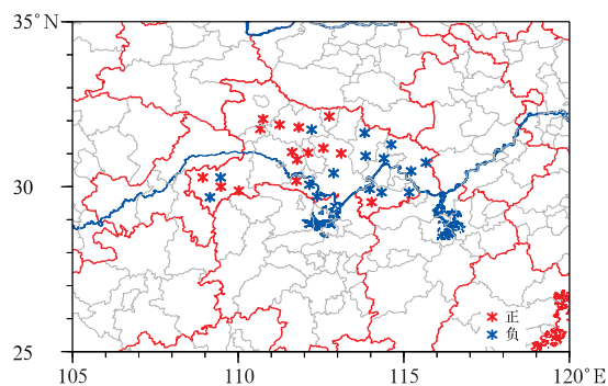
图 13 2016 年 6 月 30 日 17 时三种云微物理方案模拟的大气可降水量与观测的差值分布
