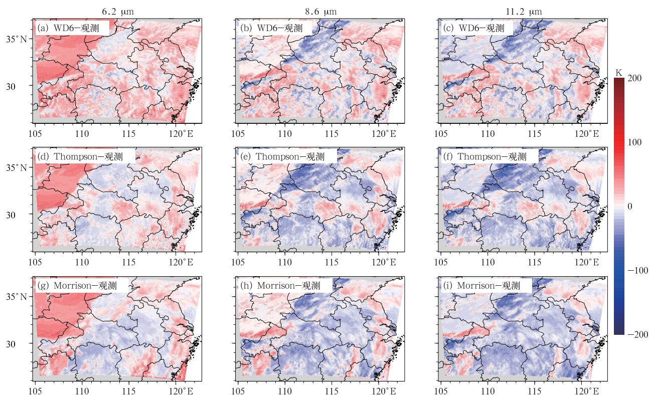
图 10 2016 年 6 月 30 日 18 时三个通道三种云微物理方案模拟与葵花 8 卫星观测的亮温差值分布
