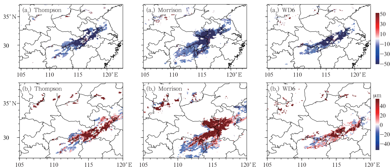
图 12 2016 年 7 月 1 日 07 时三种云微物理方案模拟的
