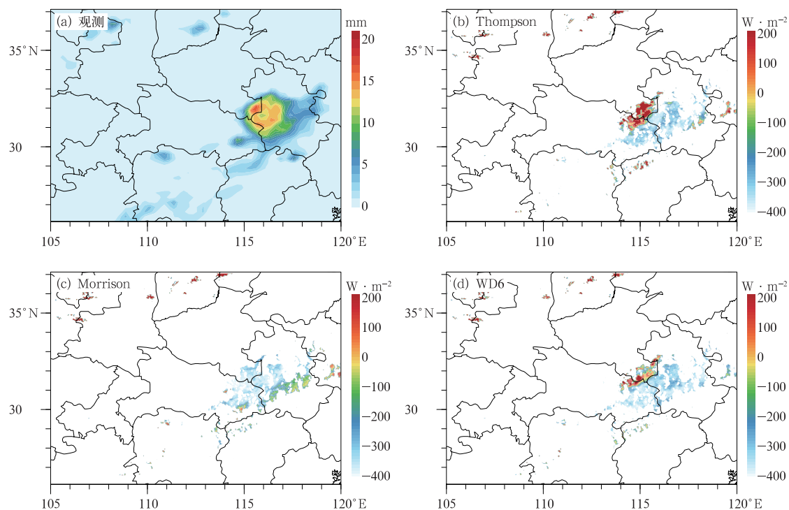
图 11 2016 年 7 月 1 日 07 时 (a) 降水量观测, (b~d) 模拟下行短波辐射与观测的差值分布
