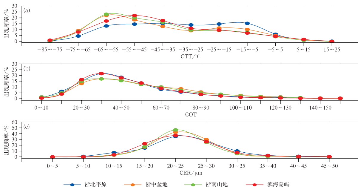
图 2 2020—2022 年夏季浙江省不同地区降水出现频率随 FY-4A 云参数的变化
