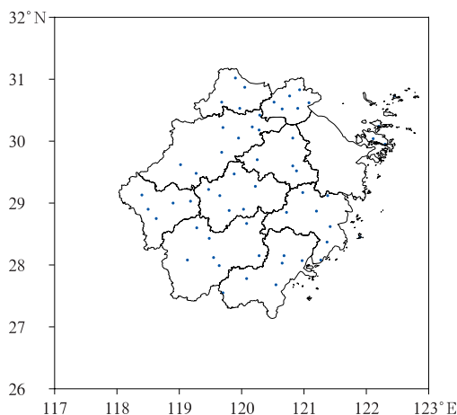
图 1 浙江省地面激光粒子谱测量仪分布
