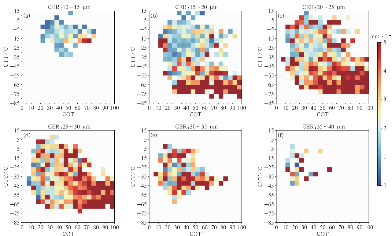
图 5 不同 CTT、COT、CER 下的降水强度中值分布
