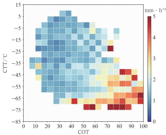
图 4 不同 CTT、COT 下的降水强度中值分布 Fig. 4 Distribution of median precipitation intensity under the collaborative influence of CTT and COT
