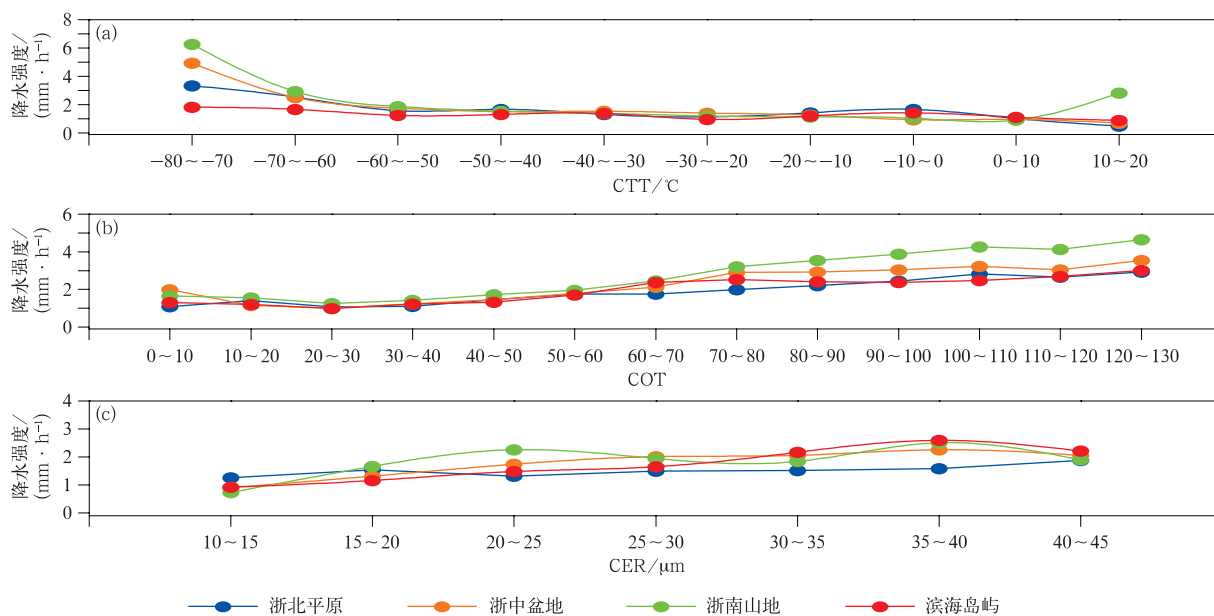
图 3 2020—2022 年夏季浙江省不同地区降水强度随 FY-4A 云参数的变化
