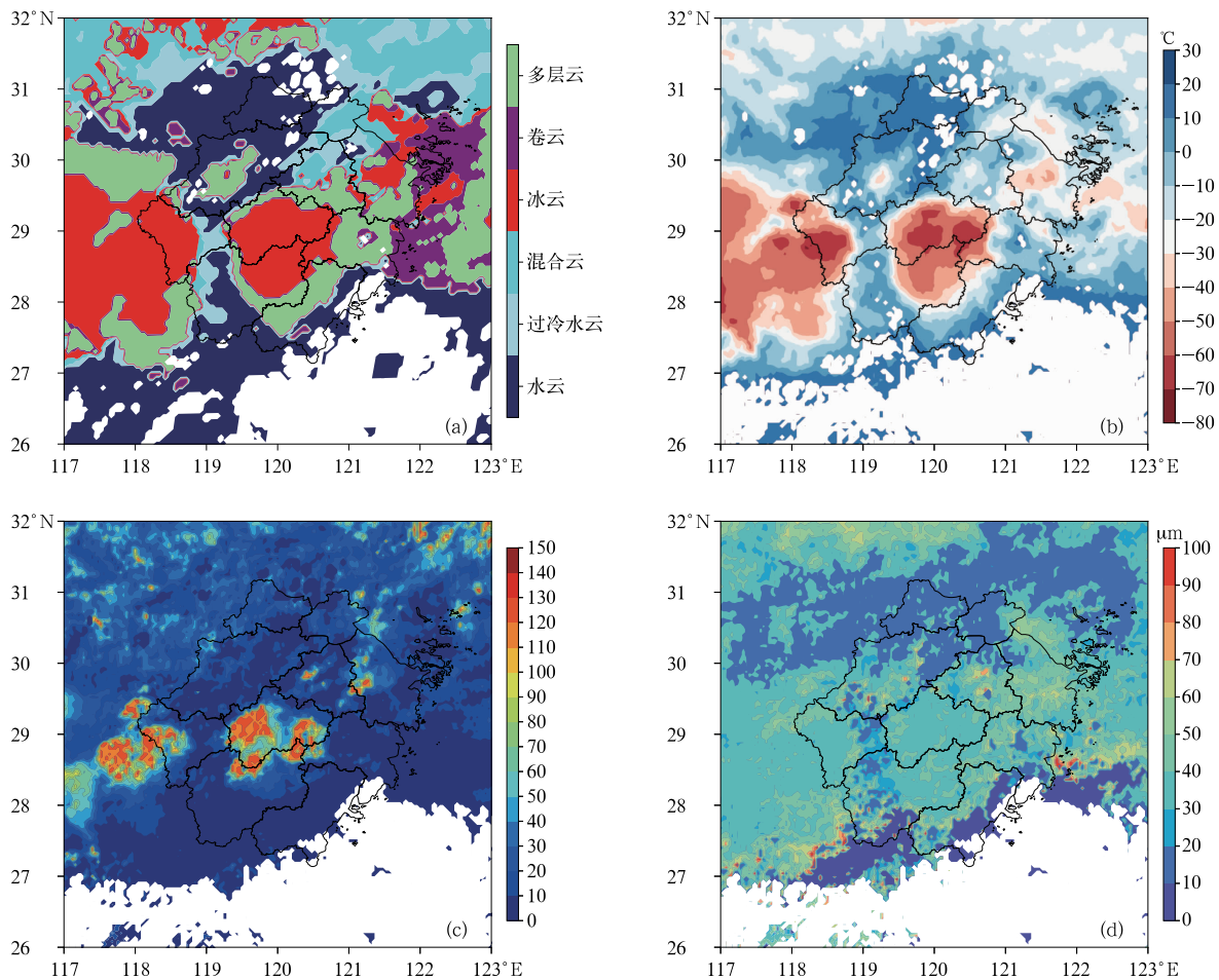
图 9 2023 年 6 月 5 日 16 时浙江省 (a)CLT, (b)CTT, (c)COT, (d)CER
