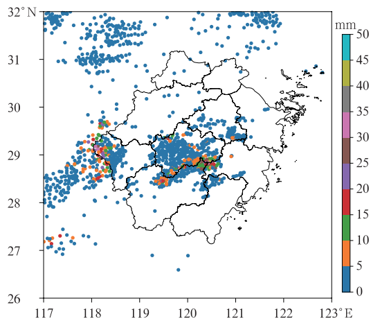
图 10 2023 年 6 月 5 日 16—17 时 浙江省降水量
