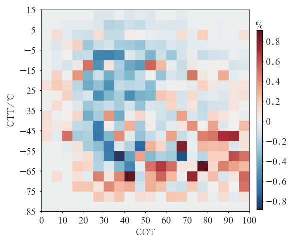
图 8 不同 CTT、COT 下的对流云和 层状云降水出现频率的差值分布
