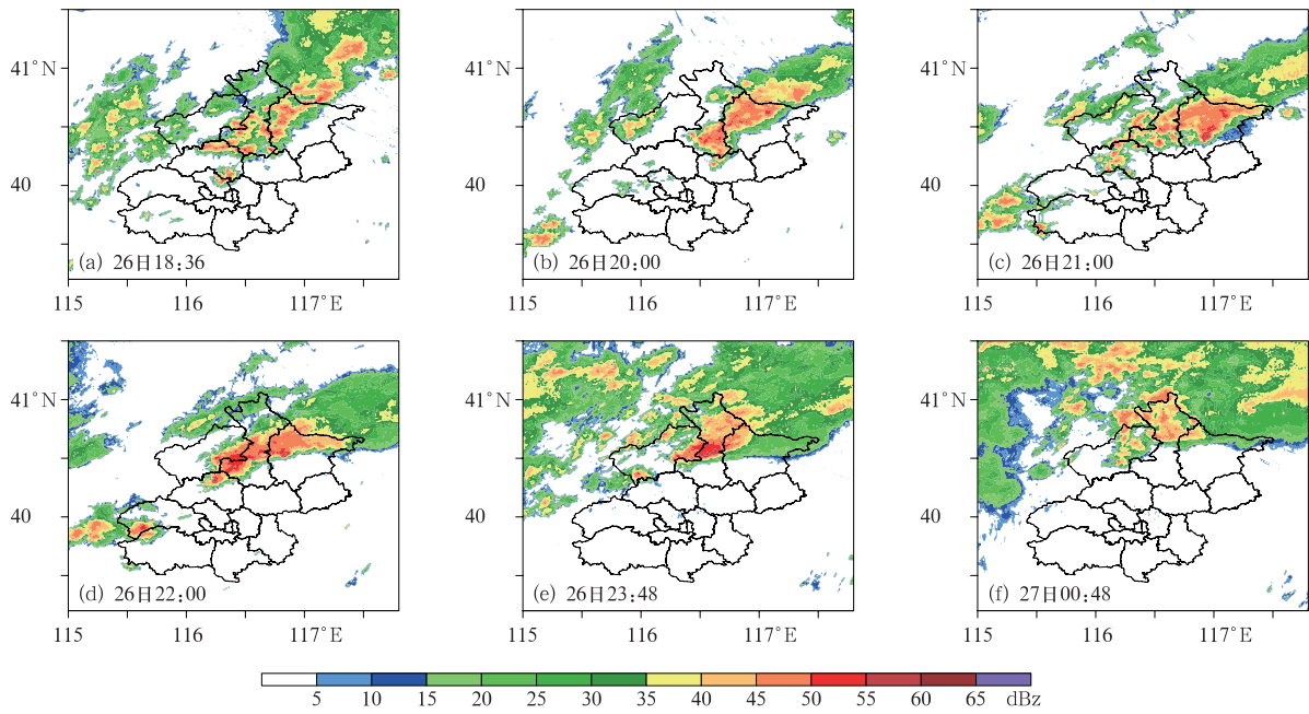
图 6 2025 年 7 月 26—27 日雷达组合反射率因子演变
