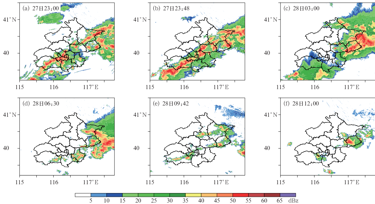
图 8 2025 年 7 月 27—28 日雷达组合反射率因子演变
