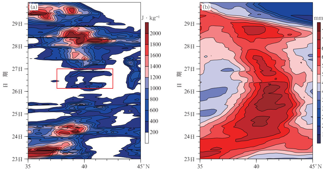
注:图 a 中红框内参照实况探空进行订正。
