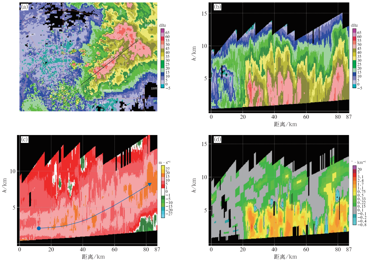
图 9 2025 年 7 月 28 日 03:00 北京气象台雷达(a)组合反射率因子分布,(b)反射率因子、(c)径向速度和(d) K_{DP} 沿图 9a 中黑线的垂直剖面
