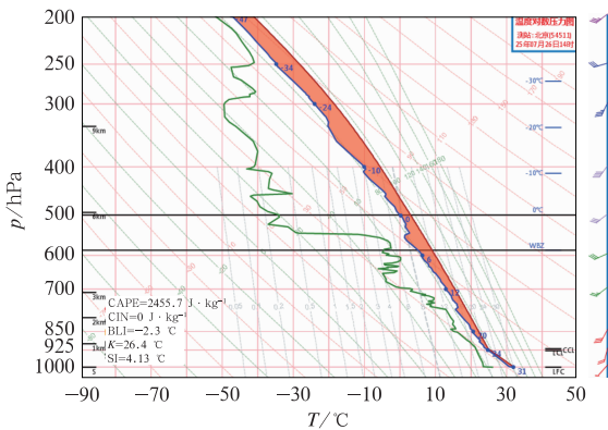
图 12 2025 年 7 月 26 日 14:00 北京气象台探空曲线 Fig. 12 Radiosonde observation at Beijing Observatory at 14:00 BT 26 July 2025
