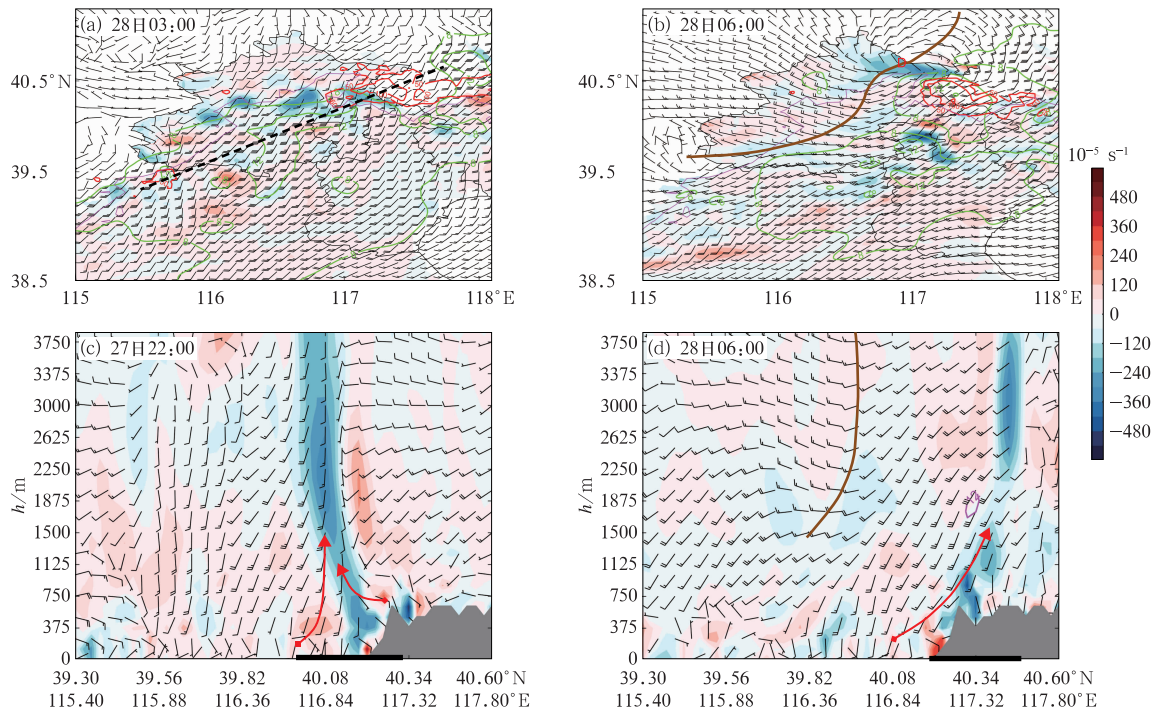
注:图 a, b 中紫红色线为 200 m 地形高度线,绿色等值线为风速 \geq 8 \text{ m} \cdot \text{s}^{-1} ,D 示意中尺度低涡; 图 c, d 中紫红色线为水平风速 \geq 12 \text{ m} \cdot \text{s}^{-1} ,灰色阴影为地形, 红色箭头线示意迎风坡附近气流辐合,横轴上黑色线段示意降水位置;棕色线为切变线。
