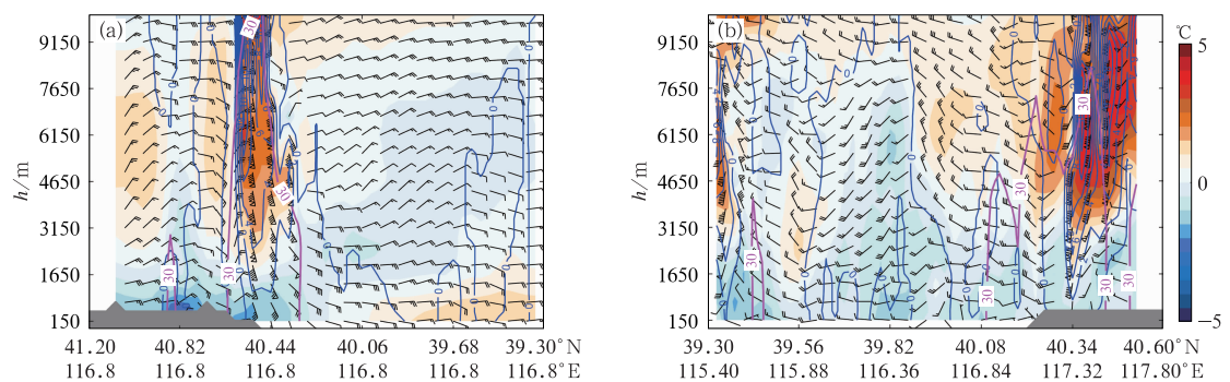
图 16 2025 年 7 月(a)26 日 20:30 沿图 14b 黑色虚线,(b)28 日 02:30 沿图 15a 黑色虚线的扰动温度(填色),30 dBz 雷达反射率因子(紫红色等值线),垂直上升速度(蓝色等值线,单位: \text{m} \cdot \text{s}^{-1} )和全风场(风羽,垂直速度扩大 10 倍)的垂直剖面
