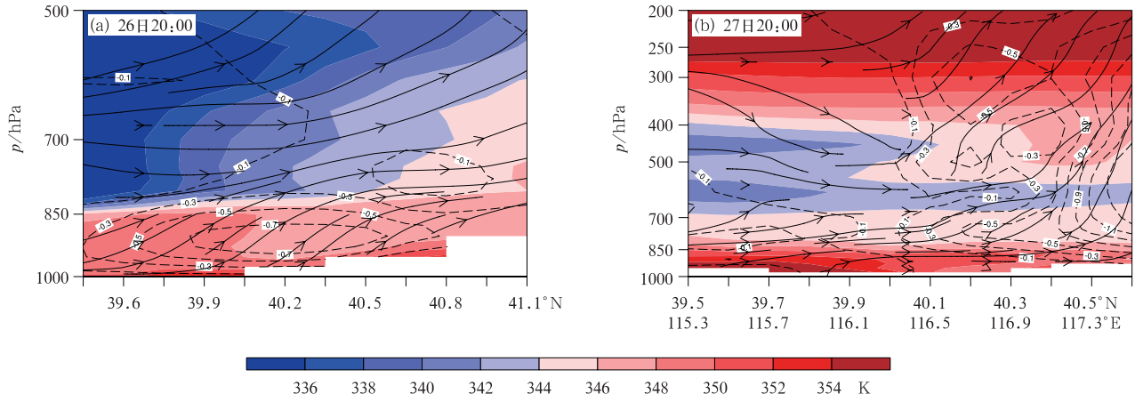
图 13 2025 年 7 月 26—27 日 (a)沿 116.8°E, (b)沿图 1 中虚线的 \theta_{se} (填色)、 流场(流线)和垂直速度(虚线,单位: \text{Pa} \cdot \text{s}^{-1} )的垂直剖面
