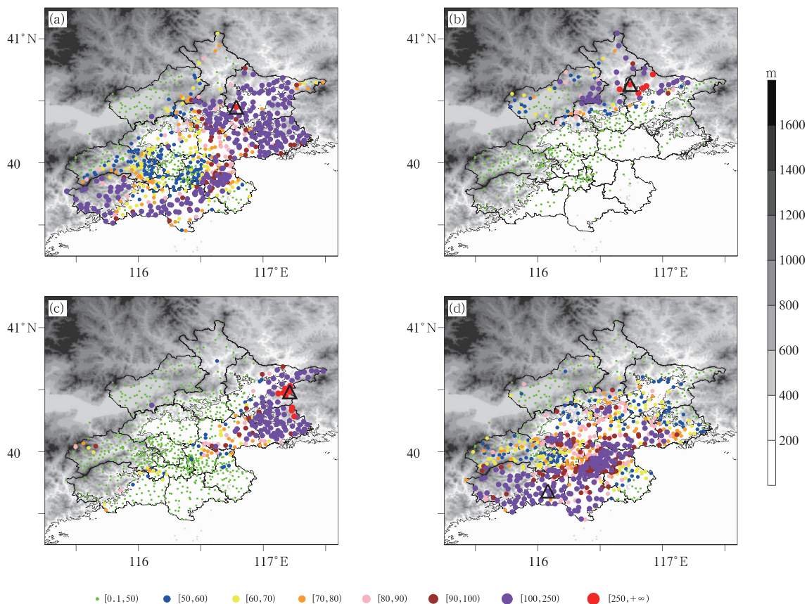
注:图中黑色三角标注各阶段最大降水量。
