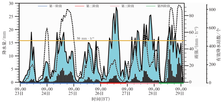
图 3 暴雨四个阶段的全市平均降水量(柱状)、有效降水站数(虚线)和单站最大雨强(实线填色)的逐时变化
