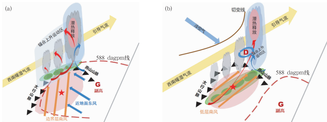
图 17 北京“25·7”极端暴雨(a)第二和(b)第三阶段概念模型
