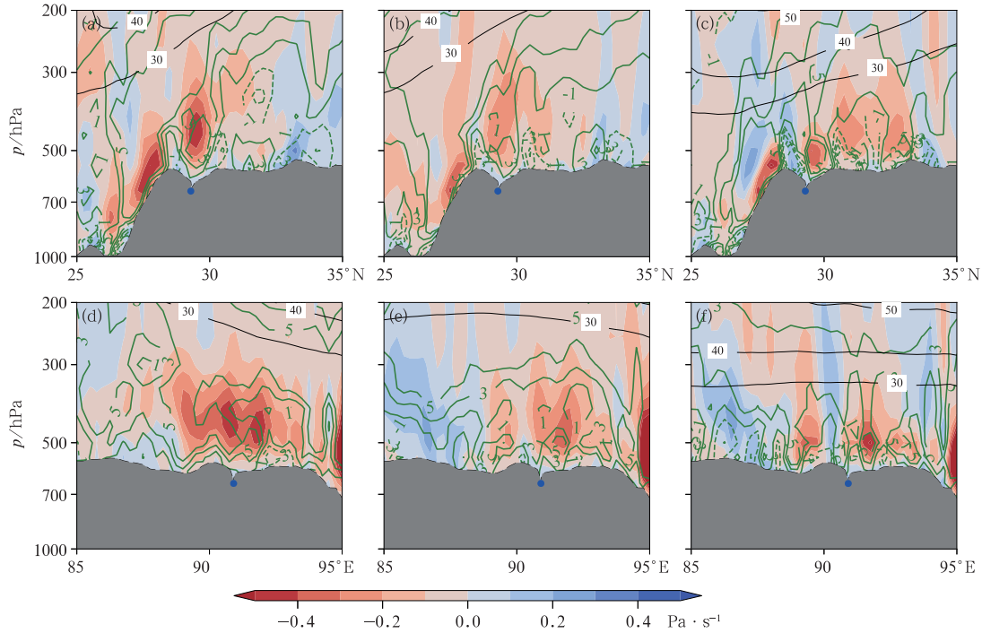
图 5 2013—2020 年拉萨机场降雪天气(a,d)气旋型,(b,e)低压槽型,(c,f)西风平流型的涡度(绿色等值线,单位: 10^{-5} \text{ s}^{-1} )、垂直速度(填色)和水平风速(黑色等值线,单位: \text{m} \cdot \text{s}^{-1} )的(a~c)经向和(d~f)纬向剖面
