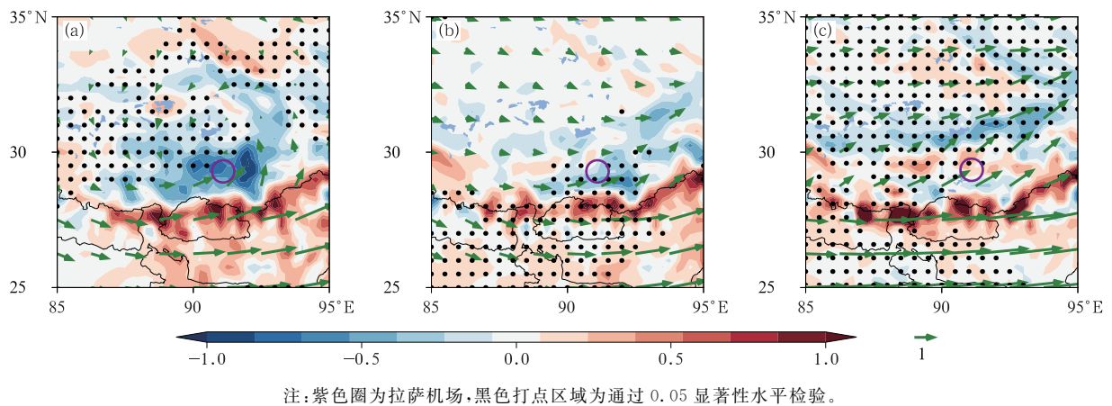
图 7 2013—2020 年拉萨机场降雪天气(a)气旋型,(b)低压槽型,(c)西风平流型 500 hPa 水汽通量(绿色箭头,单位: g \cdot cm^{-1} \cdot hPa^{-1} \cdot s^{-1} )与水汽通量散度(填色,单位: 10^{-7} g \cdot cm^{-2} \cdot hPa^{-1} \cdot s^{-1} )
