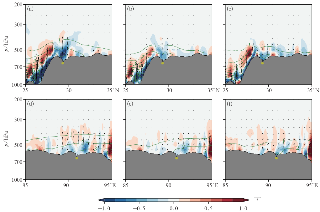
图 8 2013—2020 年拉萨机场降雪天气(a,d)气旋型,(b,e)低压槽型,(c,f)西风平流型水汽通量(箭头,单位: \text{g} \cdot \text{cm}^{-1} \cdot \text{hPa}^{-1} \cdot \text{s}^{-1} )、水汽通量散度(填色,单位: 10^{-7} \text{ g} \cdot \text{cm}^{-2} \cdot \text{hPa}^{-1} \cdot \text{s}^{-1} )和比湿(绿色等值线,单位: \text{g} \cdot \text{kg}^{-1} )的(a~c)经向和(d~f)纬向剖面
