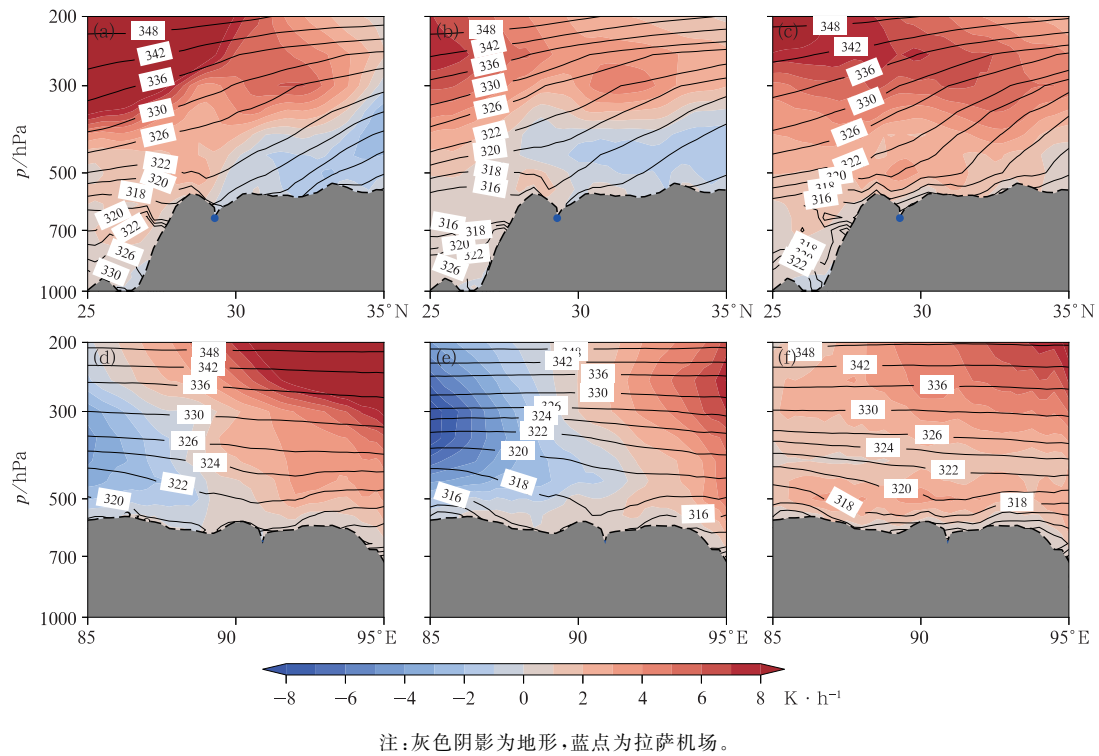
图 6 2013—2020 年拉萨机场降雪天气(a,d)气旋型,(b,e)低压槽型,(c,f)西风平流型相当位温(等值线,单位:K)和温度平流(填色)的(a~c)经向和(d~f)纬向剖面
