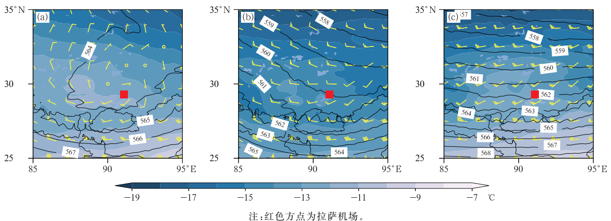
图 3 2013—2020 年拉萨机场降雪天气(a)气旋型,(b)低压槽型,(c)西风平流型的 500 hPa 位势高度场(等值线,单位:dagpm)、温度场(填色)与风场(风羽)
