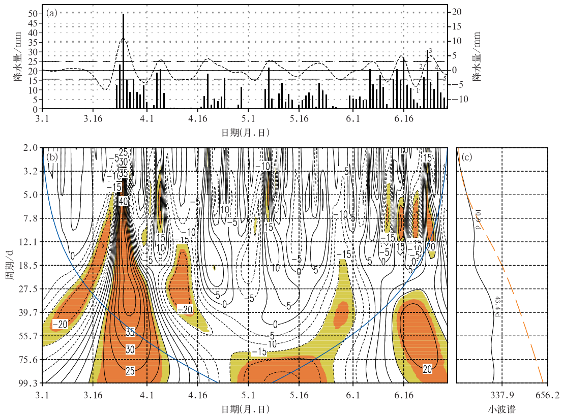
注:图 a 中上下两条水平虚线表示 7~20 d 滤波降水的一倍标准差,1~5 分别为 5 个位相;图 b 中黄色和棕色分别表示通过 0.1 和 0.05 显著性水平检验的区域,两侧蓝色的弧线下区域表示边界效应的影响域;图 c 中棕色虚线为 0.1 显著性水平线。显著性水平检验采用了 Monte-Carlo 方法。
