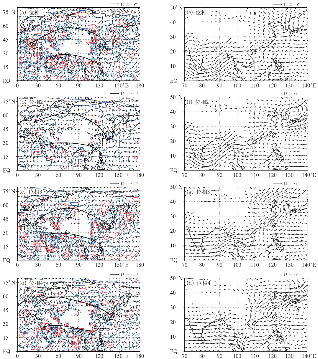
注:“A”和“C”分别代表异常反气旋和异常气旋,黑弧线表示波列。
