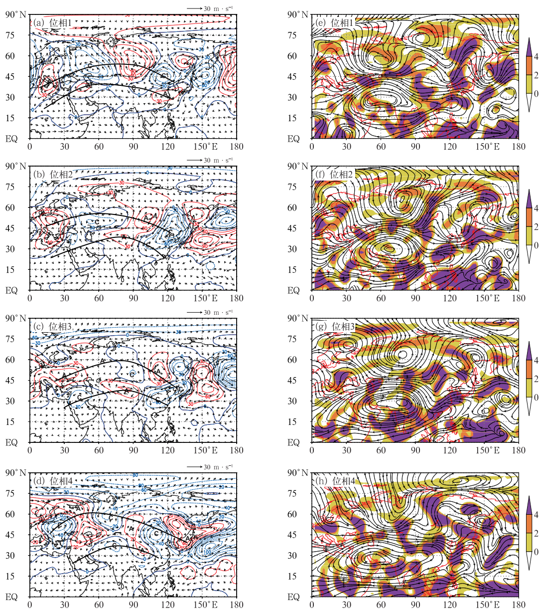
注:图 a~d 中“A”和“C”分别代表异常反气旋和异常气旋;黑弧线表示波列。
