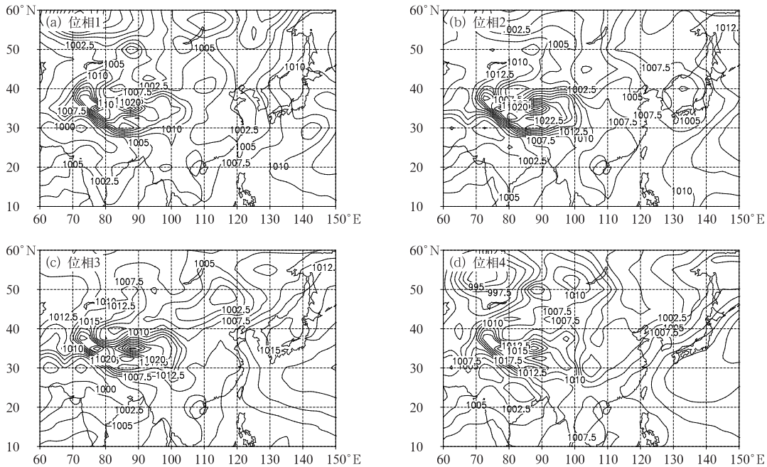
图 8 2023 年 6 月 22—26 日广东连续暖区暴雨过程位相 1~4 的海平面气压场分布(单位:hPa)
