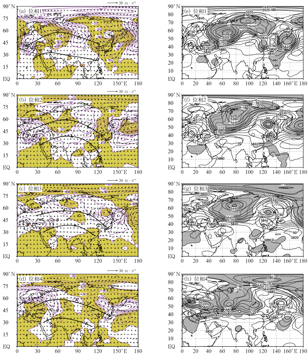
注:图 a~d 中“A”和“C”分别代表异常反气旋和异常气旋,黑弧线表示波列。
