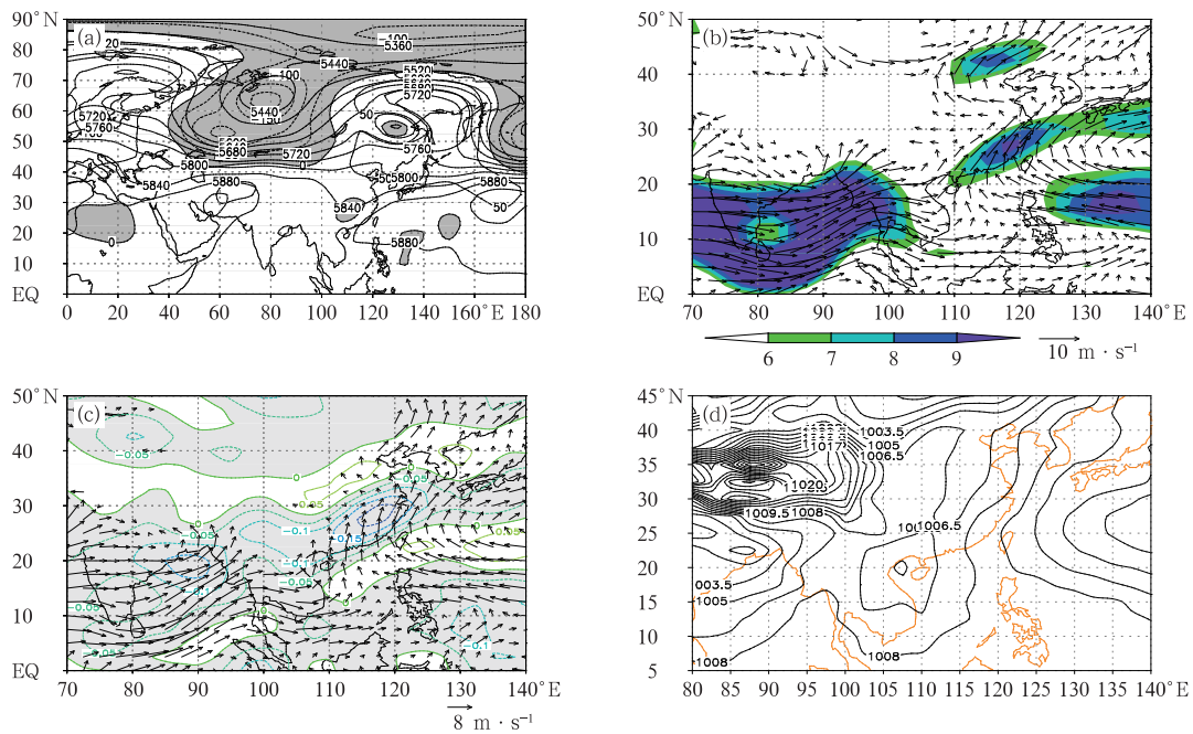
图 4 2023 年 6 月 22—26 日广东连续暖区暴雨过程平均的(a)500 hPa 高度场(实线,单位:gpm)及其距平场(虚线,阴影区为负距平,单位:gpm), (b)850 hPa 风场(箭头)及风速(填色,单位: \text{m}\cdot\text{s}^{-1} ), (c)925 hPa 风场(箭头)、500 hPa 垂直速度(等值线,阴影表示负值,单位: \text{hPa}\cdot\text{s}^{-1} ), (d)海平面气压场(单位:hPa)
