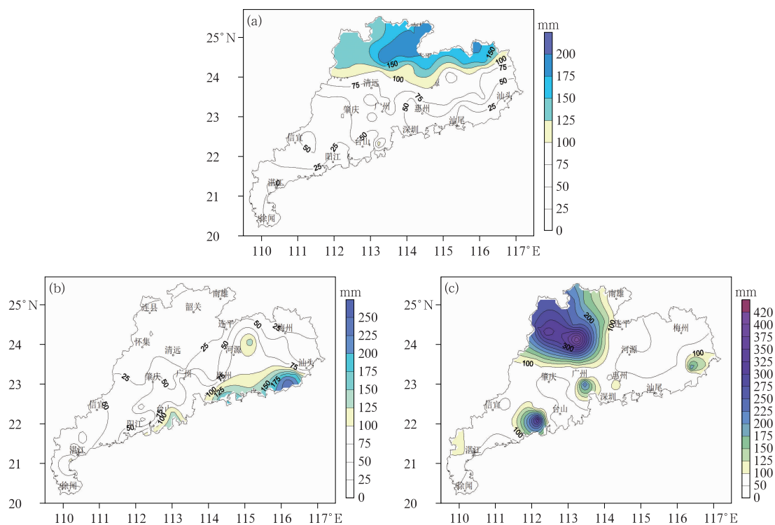
图 2 2023 年(a)3 月 23—25 日,(b)6 月 14—16 日,(c)6 月 22—26 日广东三次连续暴雨过程累计降水量 Fig. 2 The accumulated precipitation of three continuous rainstorms in Guangdong Province during (a) 23—25 March, (b) 14—16 June and (c) 22—26 June 2023
